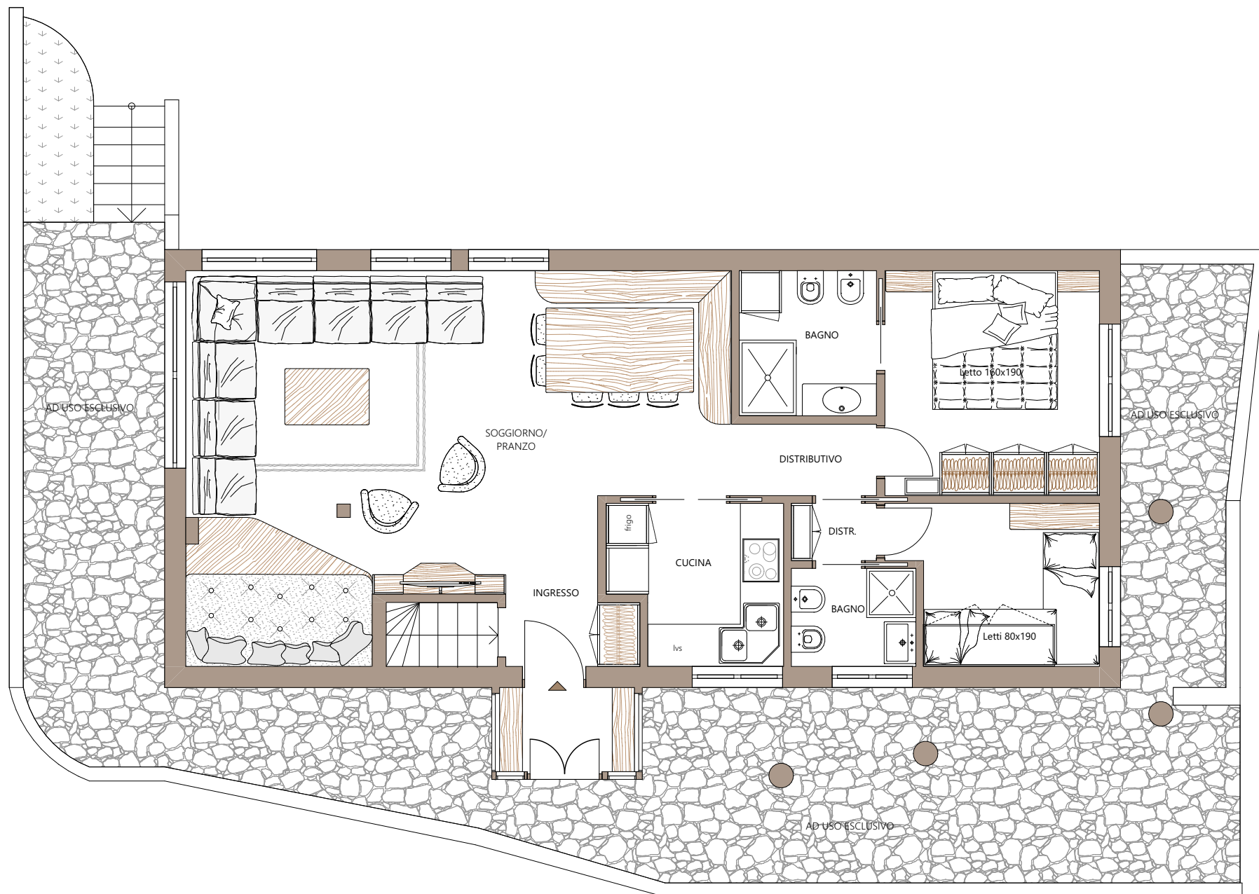
Planimetria Stato di progetto Piano Terra
